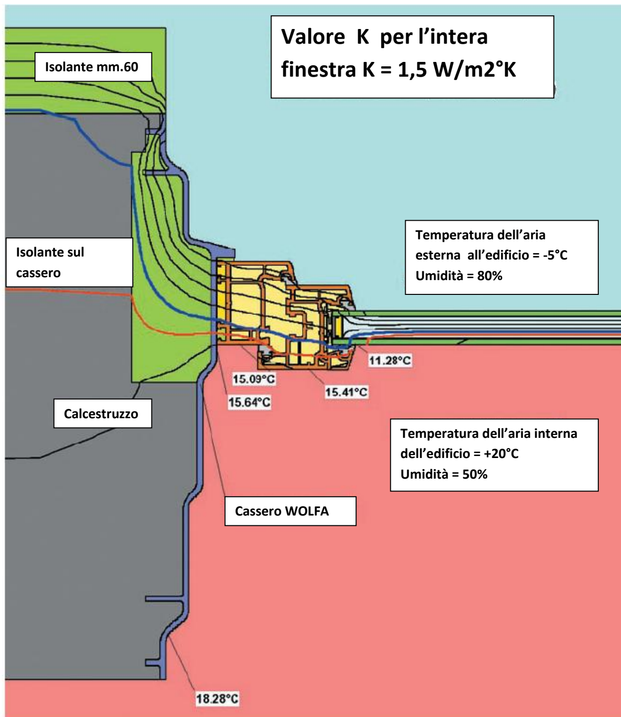
FINESTRA WOLFA MODELLO DK – VETRO ISOLANTE DA 24 MM.
